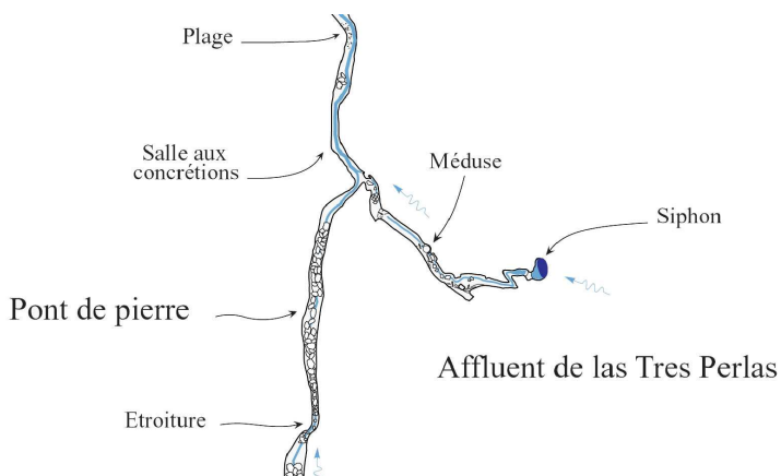
Fig. 4 : Plan de l'affluent des Trois Perles.
